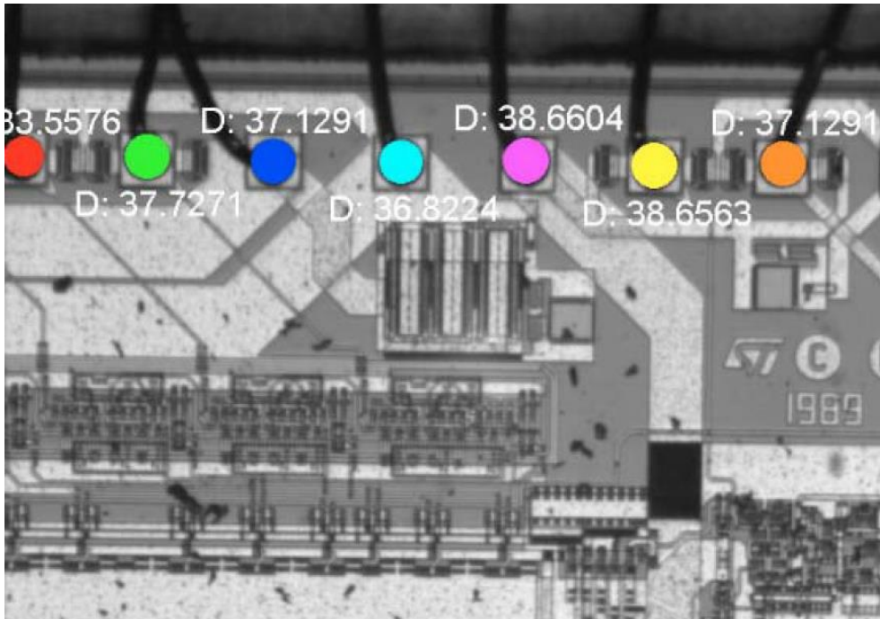
그림) 볼 본드 직경의 자동 측정
