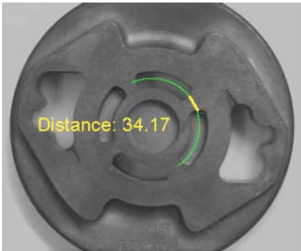
그림) 주물 구멍 사이의 거리를 자동으로 측정
