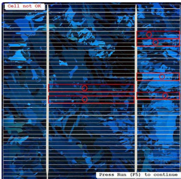
그림) 태양 전지의 결함이 있는 핑거 추출
